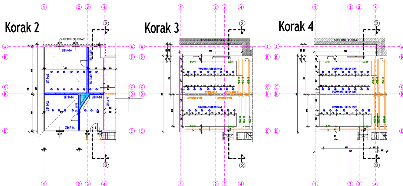
Slika 8 deo postupaka predloženih mera sanacije „levog“ dela kuće
