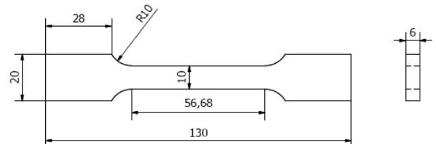
Slika 8 – Dimenzije epruvete za ispitivanje na zatezanje
