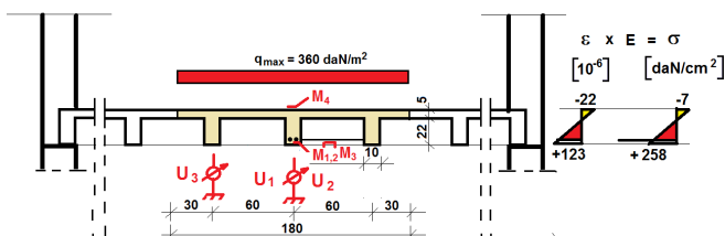
Slika 5: Dijagrami merenih dilatacija i napona u armaturi i betonu
